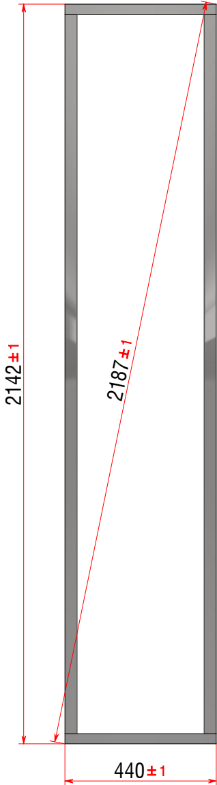
FRENTE ( 1 : 15 )
